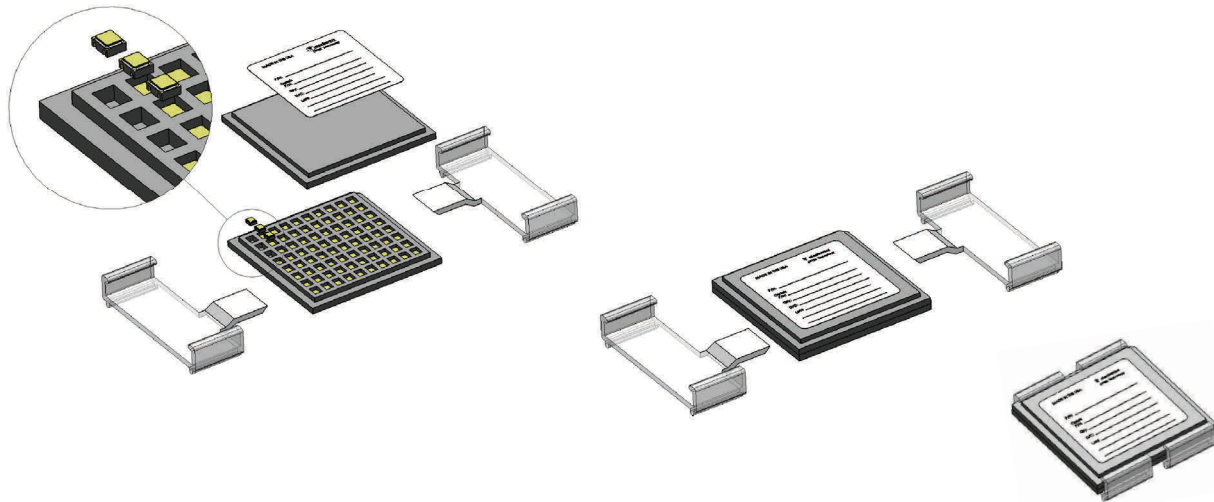
Waffle Pack
