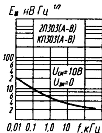
Зависимость ЭДС шума от частоты
