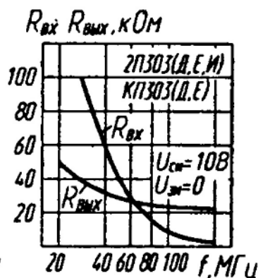
Зависимости входного и выходного сопротивлений от частоты
