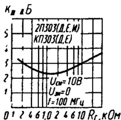
Зависимость коэффициента шума от сопротивления генератора
